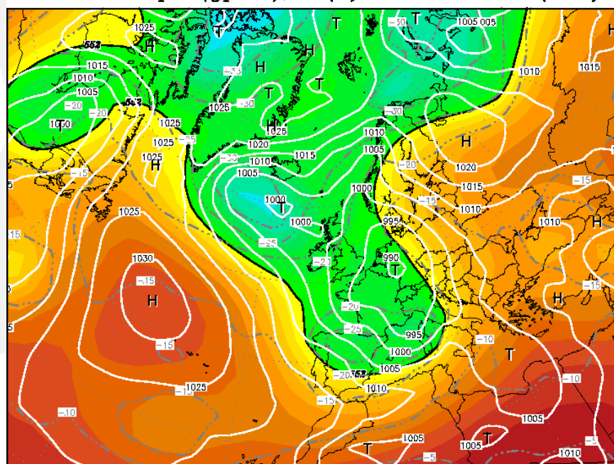
Figura 1: il modello previsionale GFS indica il passaggio di un fronte freddo previsto per il giorno 17 maggio.
